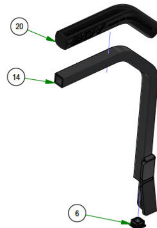
031-9071-00 LEFT HAND DRIVE ARM
