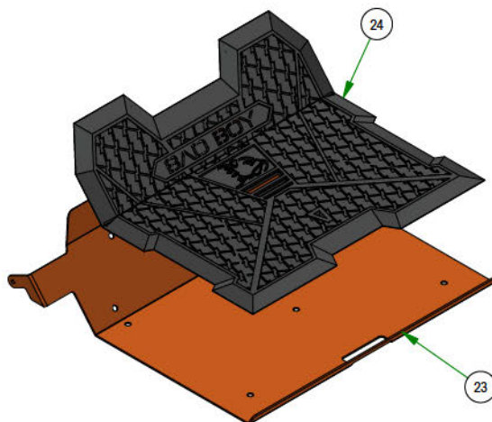
079-3155-24 FLOORBOARD ASSEMBLY
