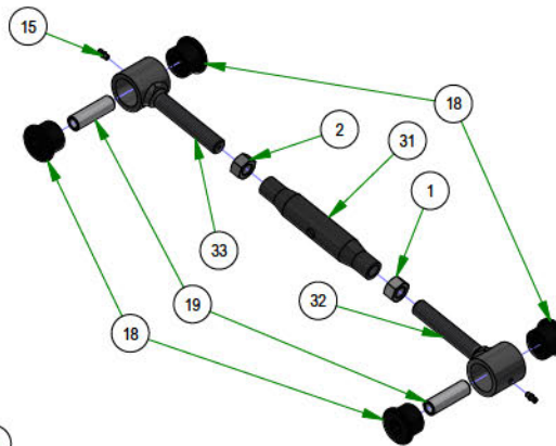
048-9000-00 TURNBUCKLE
