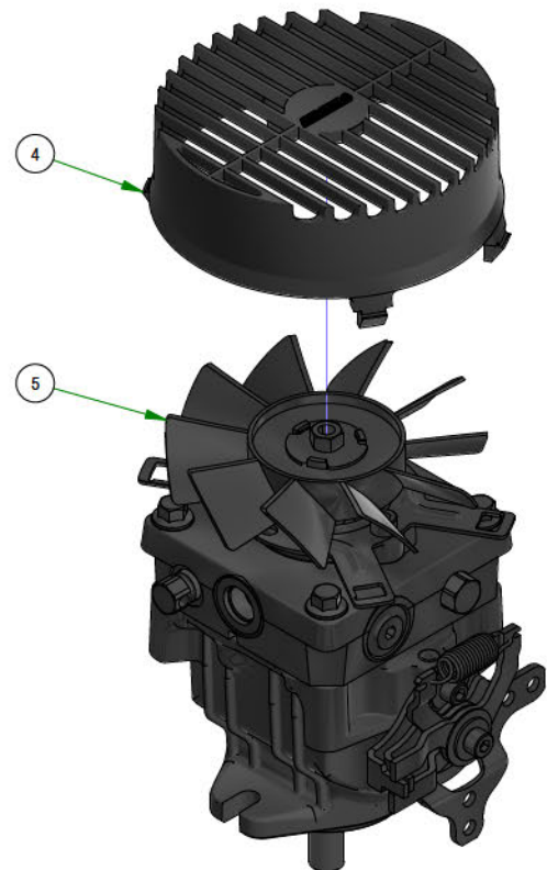
050-3001-00 & 050-3003-00 RIGHT/LEFT PUMP 16CC
