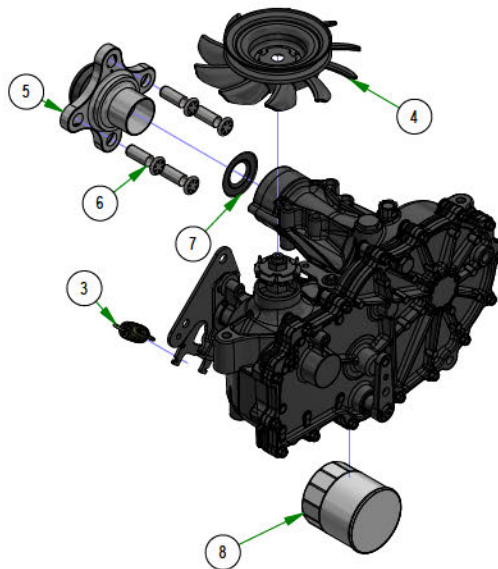
050-5050-02 2021 RH 2800 Transaxle
