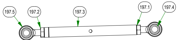
048-6061-00 UPPER RADIUS ROD
